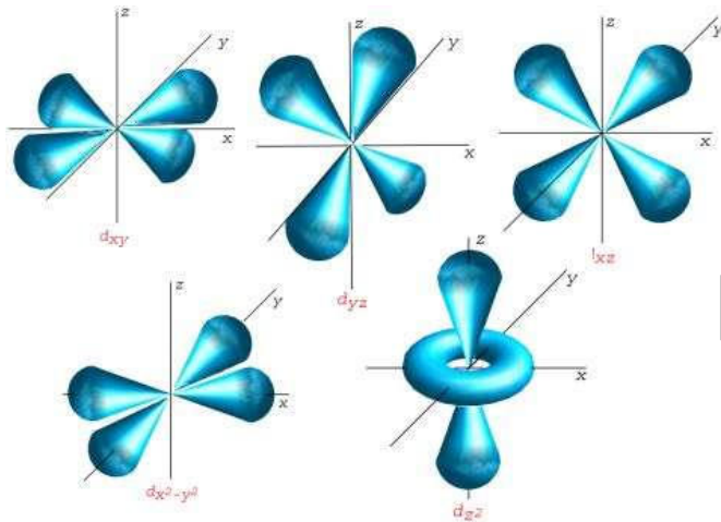
ORBITALES D
